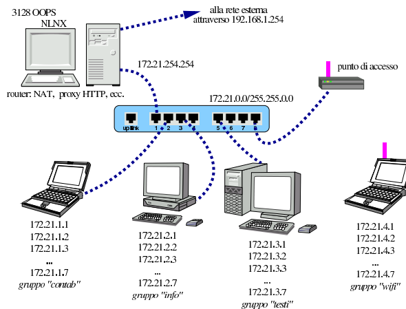
Figura u34.1. Situazione tipica di utilizzo del servizio proxy HTTP di NLNX
