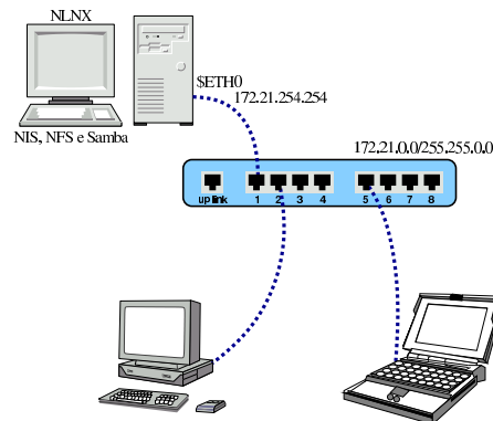
Figura u33.1. NIS, NFS e Samba offerti da un elaboratore in cui è installato NLNX.
