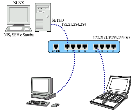
Figura u33.5. NIS, SSH e Samba offerti da un elaboratore in cui è installato NLNX.
