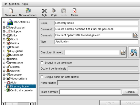
Figura 28.130. Kmenuedit.
